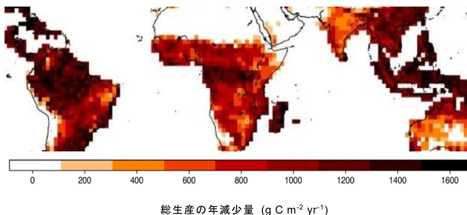
図 3. モデル計算で得られた世界の熱帯・亜熱帯林の総生産の減少度合 リンにより光合成が制限される現象をモデルに組み込んだ際に、濃い色の地域ほど総生産量が減少すると予測されています。
