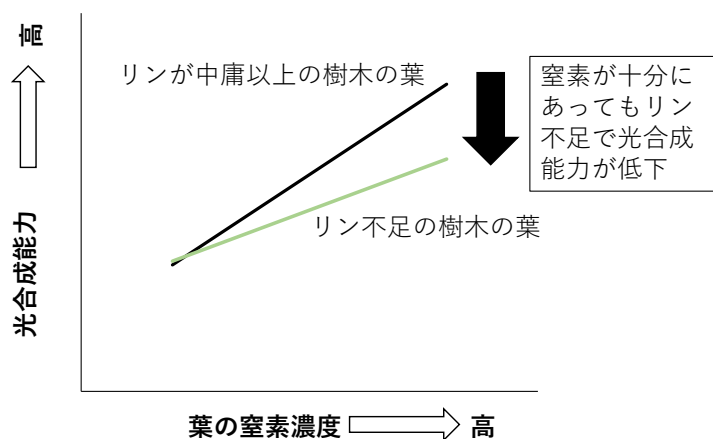
図 2. リン不足の葉とリンが不足していない葉の光合成能力の模式図 リンが不足すると、窒素が豊富にあっても光合成能力*が低下していました。この現象をモデルに組み込むことで、リン制限の定量化が可能になりました。 *ここでは最大電子伝達速度を指標としています。
